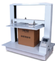
Máy kiểm tra nén
